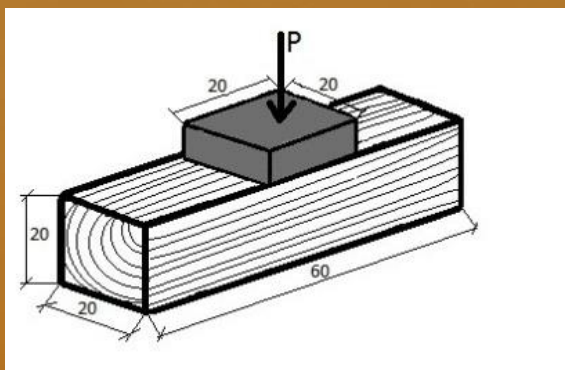
Рисунок – Внешний вид образца древесины при определении условного предела прочности при местном смятии поперек волокон
