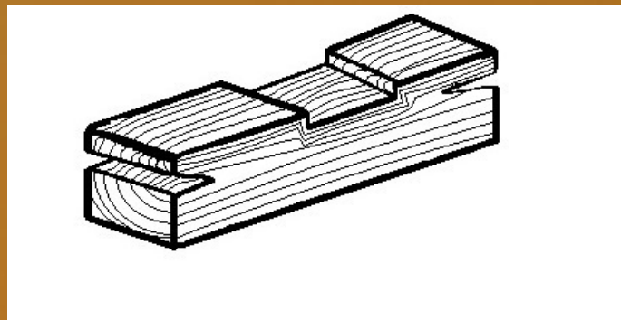
Рисунок – Внешний вид образца древесины при определении условного предела прочности при местном смятии поперек волокон
