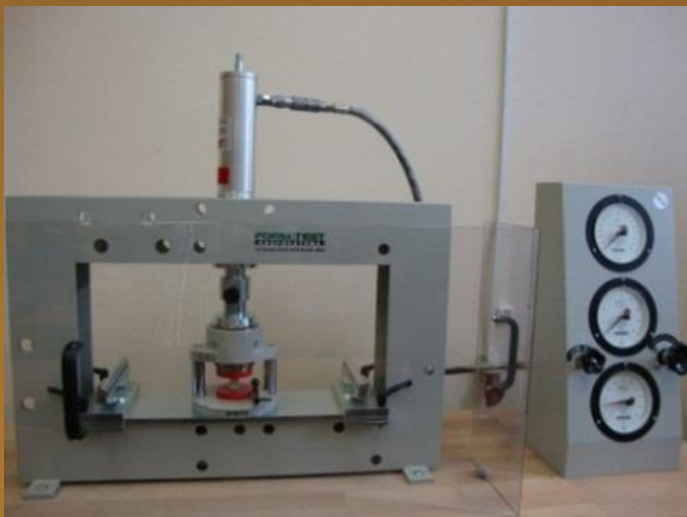
Рисунок – Определение предела прочности древесины при сжатии вдоль волокон
