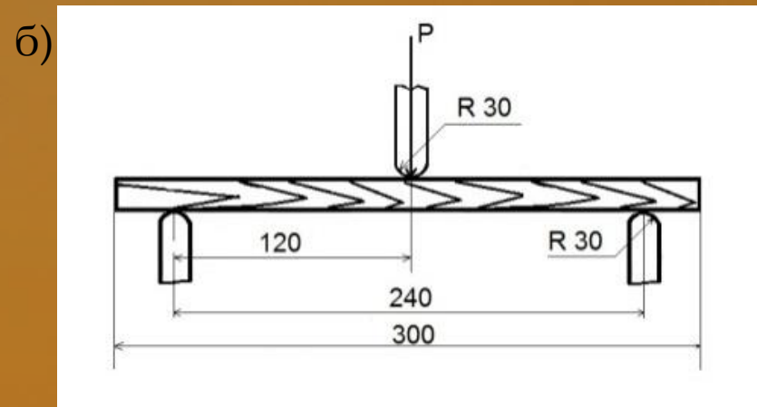
Рисунок – Испытание древесины при статическом изгибе
