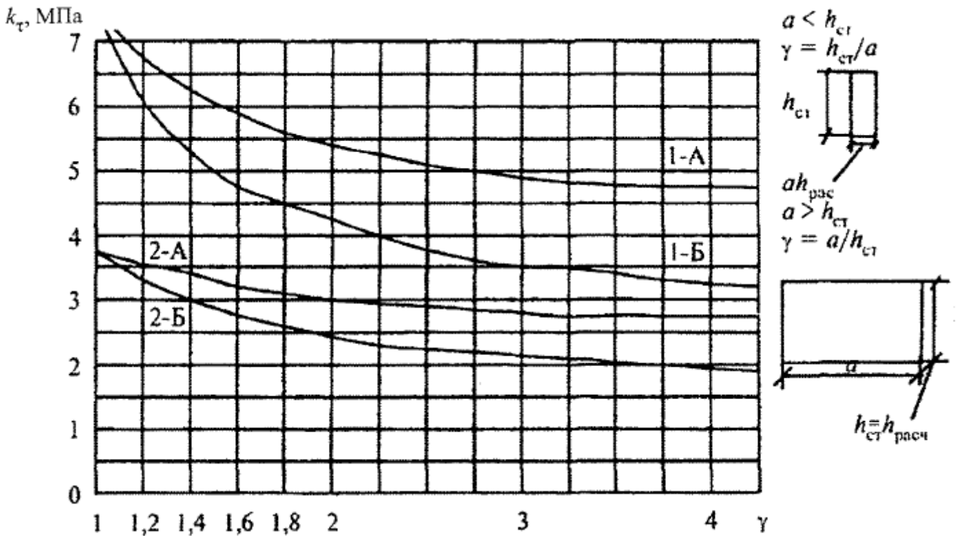
Рисунок Д.2 - Графики для определения коэффициента k_H при расположении волокон в наружных слоях фанеры вдоль пролета
