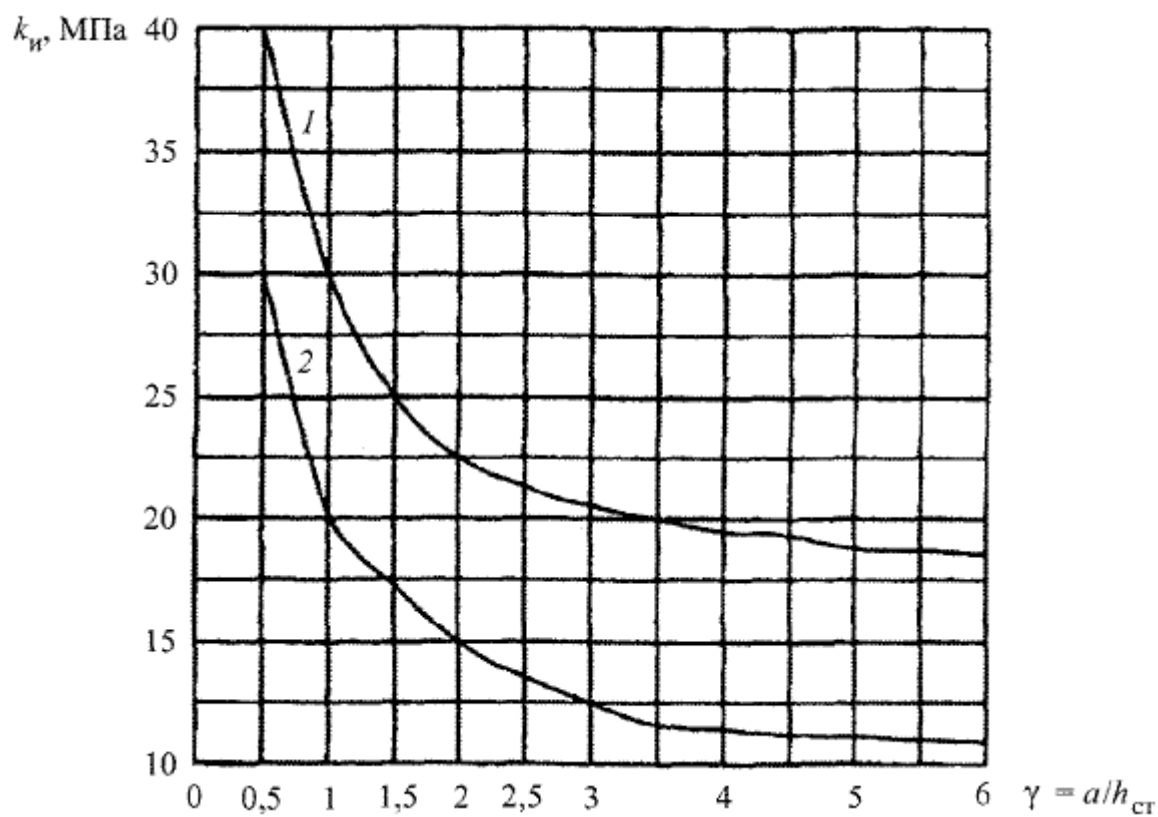
Рисунок Д.1 - Графики для определения расчетных сопротивлений при растяжении под углом к волокнам наружных слоев березовой фанеры марки ФСФ
