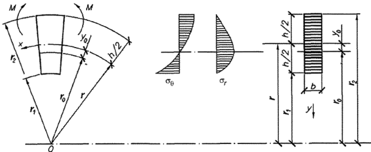
Рисунок 3 - Расчетная схема кривого бруса при чистом изгибе
