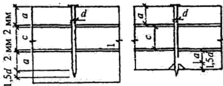
Рисунок 14 - Определение расчетной длины заземления конца гвоздя
