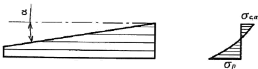
Рисунок 23 - Односкатная балка
