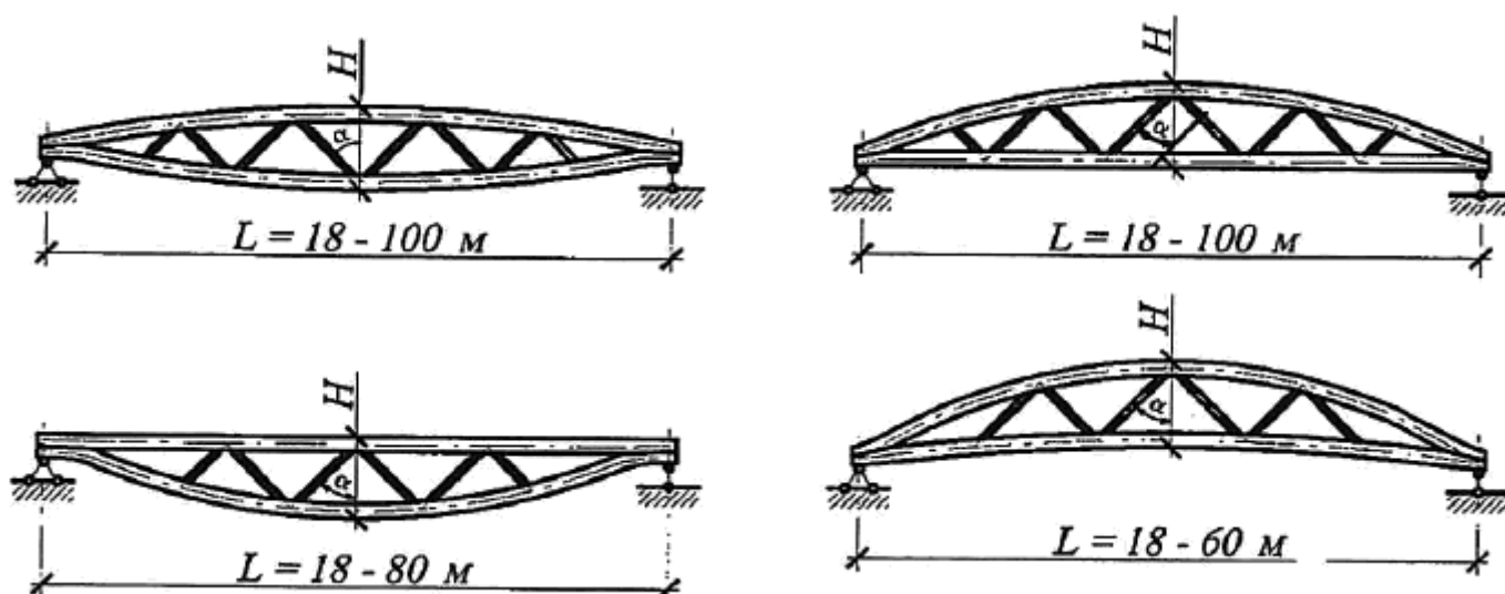
Рисунок 24 - Схемы линзообразных ферм
